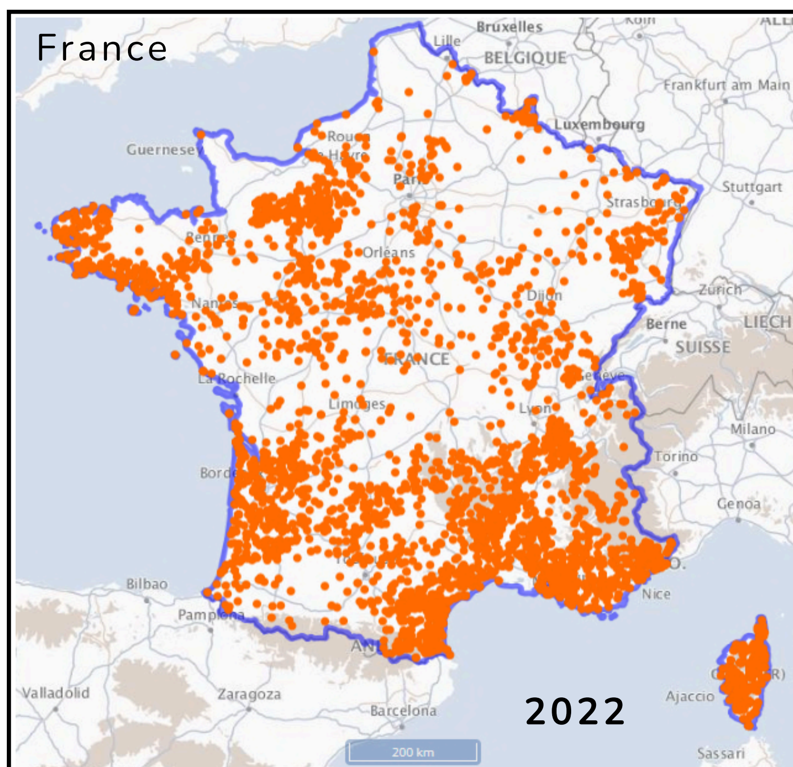
Carte des communes où au moins un incendie de forêt a été signalé (Sources : Observatoire des forêts françaises, BDIF)
